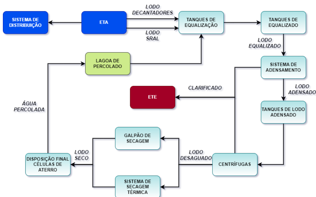
Figura 2- Fluxograma do Sistema de Adensamento, Desidratação e Secagem de Lodo.
