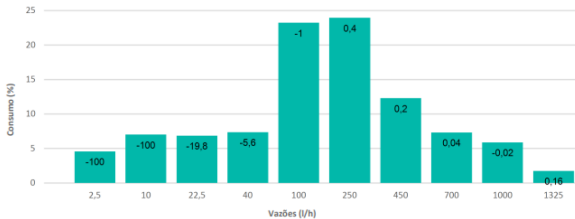
Figura 5: Histograma elaborado e função perfil típico de abastecimento domiciliar
