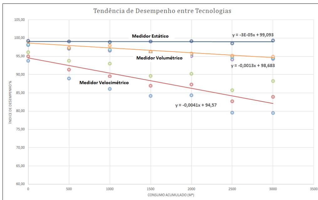
Figura 6: Tendência de desempenho metrológico–Medidor Velocimétrico x Volumétrico x Ultrassônico
