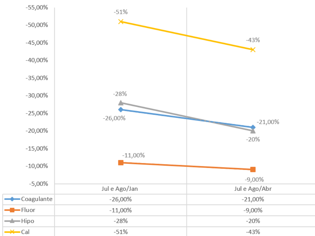
Figura 5 – Redução de produtos químicos kg/m³
